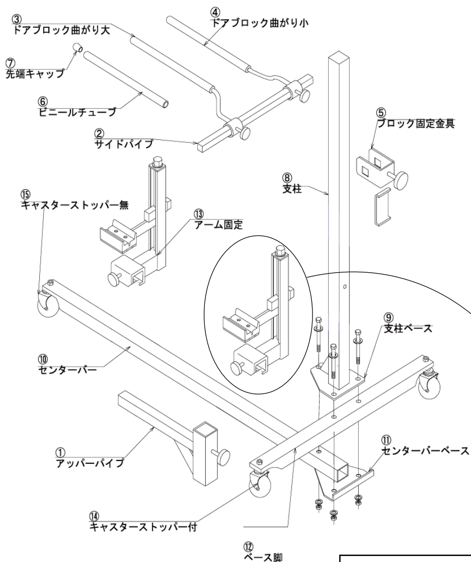
ドアリリースアーム部分解図
