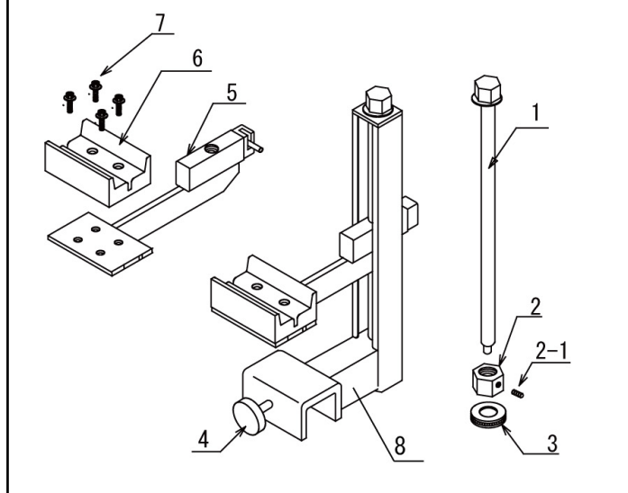
ドアリリースアーム部分解図
